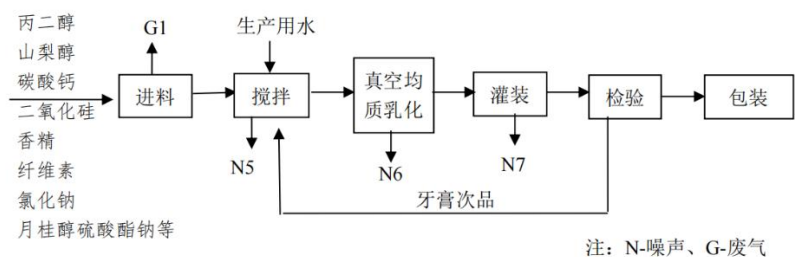
图 3.1 生产工艺流程
